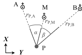
Abb. 10.53b Rückwärtseinschnitt
