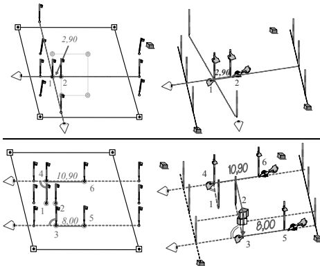
Abb. 10.64c Winkelabsteckung
