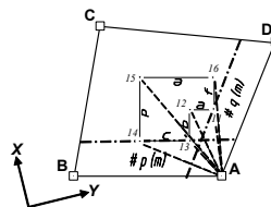
Abb. 10.67a Planungsdaten einer Gebäudeabsteckung
