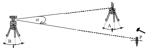
Abb. 10.64c Winkelabsteckung
