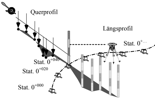
Abb. 10.58b Längs- und Querprofilaufnahme
